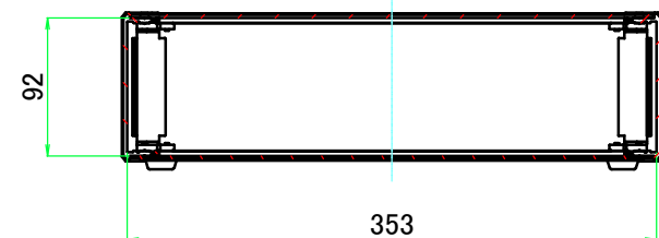
B-B ( 1 : 5.5 )
